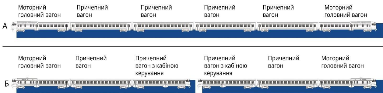
Рис. 2. Компоновка складу дизель-поїзда ДР-1А:
