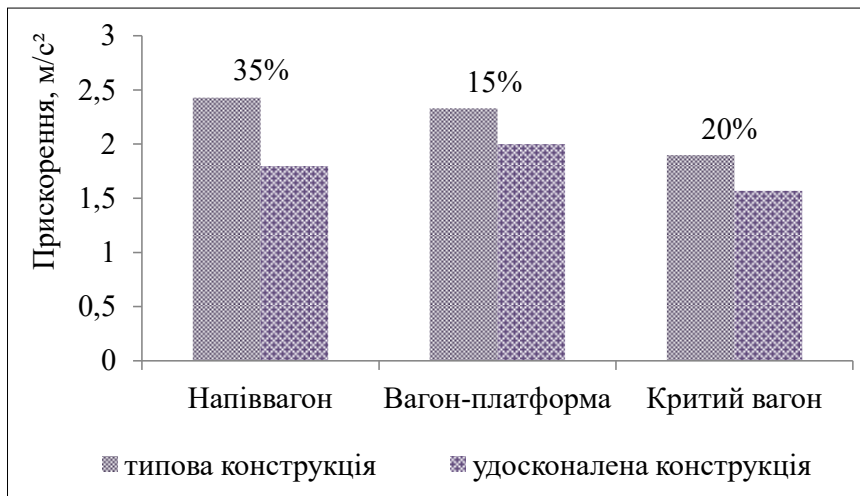
Рис. 8. Порівняльний аналіз прискорень несучих конструкцій вагонів
