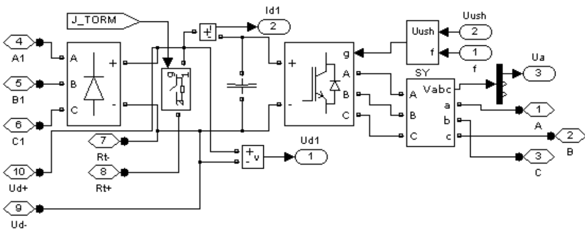
Рис.3 Модель тягового перетворювача частоти
