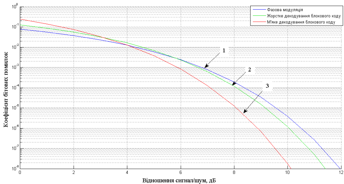
Рис. 12. Залежність ймовірності помилок від відношення сигнал/шум для двійкової фазової модуляції та блокового кодування: 1 – фазова модуляція, 2 – жорстке декодування блокового коду, 3 – м'яке декодування блокового коду
