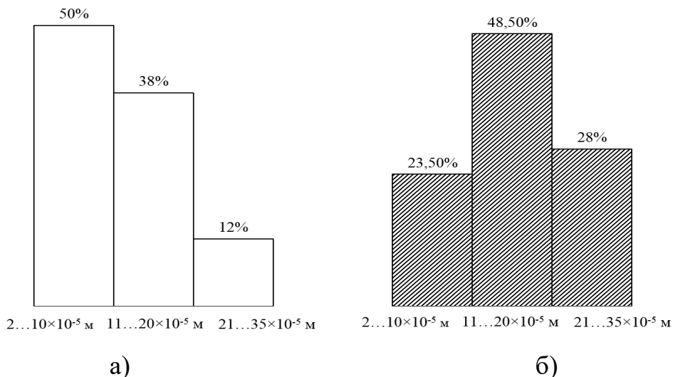
Рис. 1. Розподіл пор за розмірами, відсоток від загальної кількості: а) зразок, що містить СП, ПВД, та АМД; б) зразок, що містить СП і ПВД
